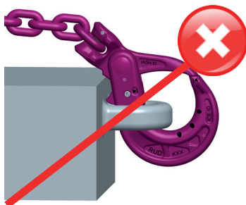
Pic. 14: No edge loading
