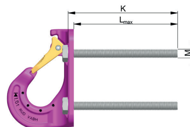
Pic. 4: bolts long (vario)
