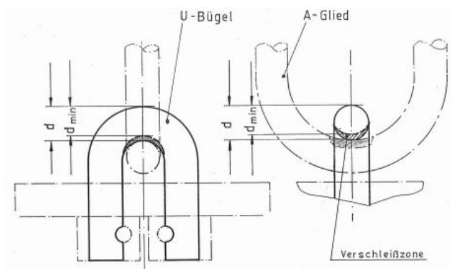
Abb. 3: Verschleißmaße
