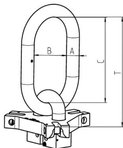
Abb. 2: Bemaßung Verteilerkopf
